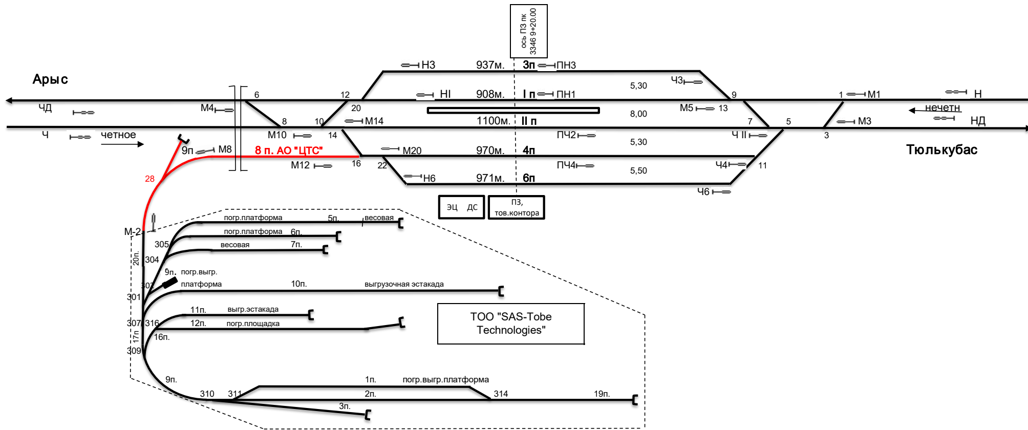
Расстояние от оси станции до постоянных сигналов и стрелок (предельных столбиков)
