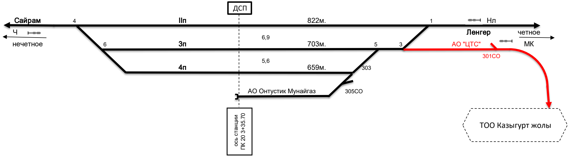
Расстояние оси ЭЦ до постоянных сигналов и стрелок (предельных столбиков)
