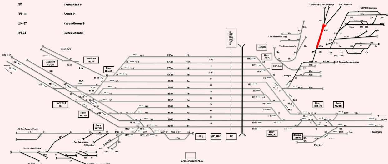
Схематический план станции Толькубас (2 класса, участковая)
